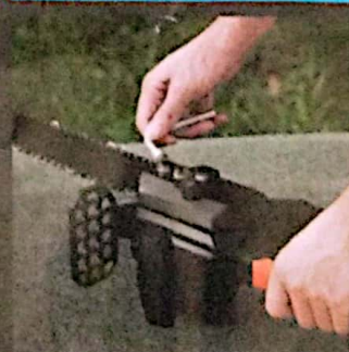
04: Coloque o pino na parte de trás da placa azul no furo fixo da placa de guia durante a instalação.
